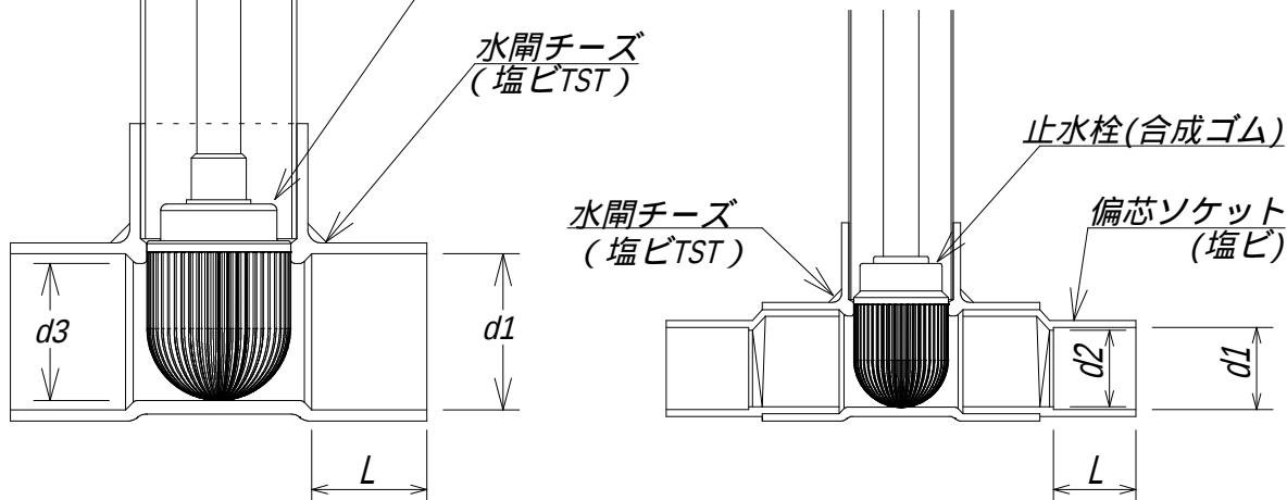
止水栓 (合成ゴム) 50 受口詳細
