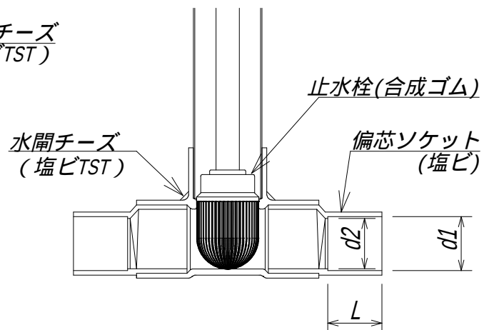
止水栓 (合成ゴム) 50 受口詳細
